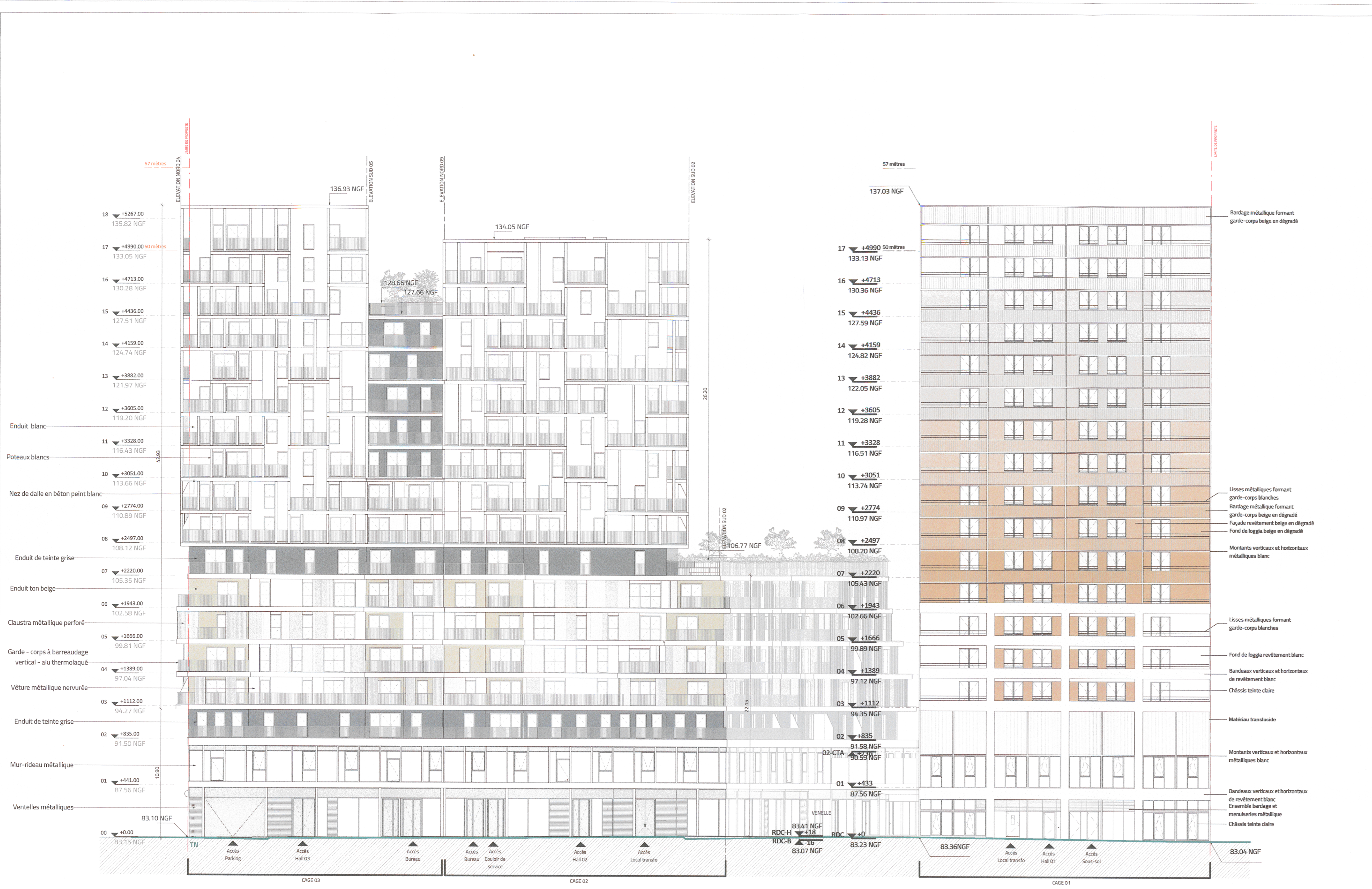
PC05a1_FACADE OUEST 01 Ech : 1:200
