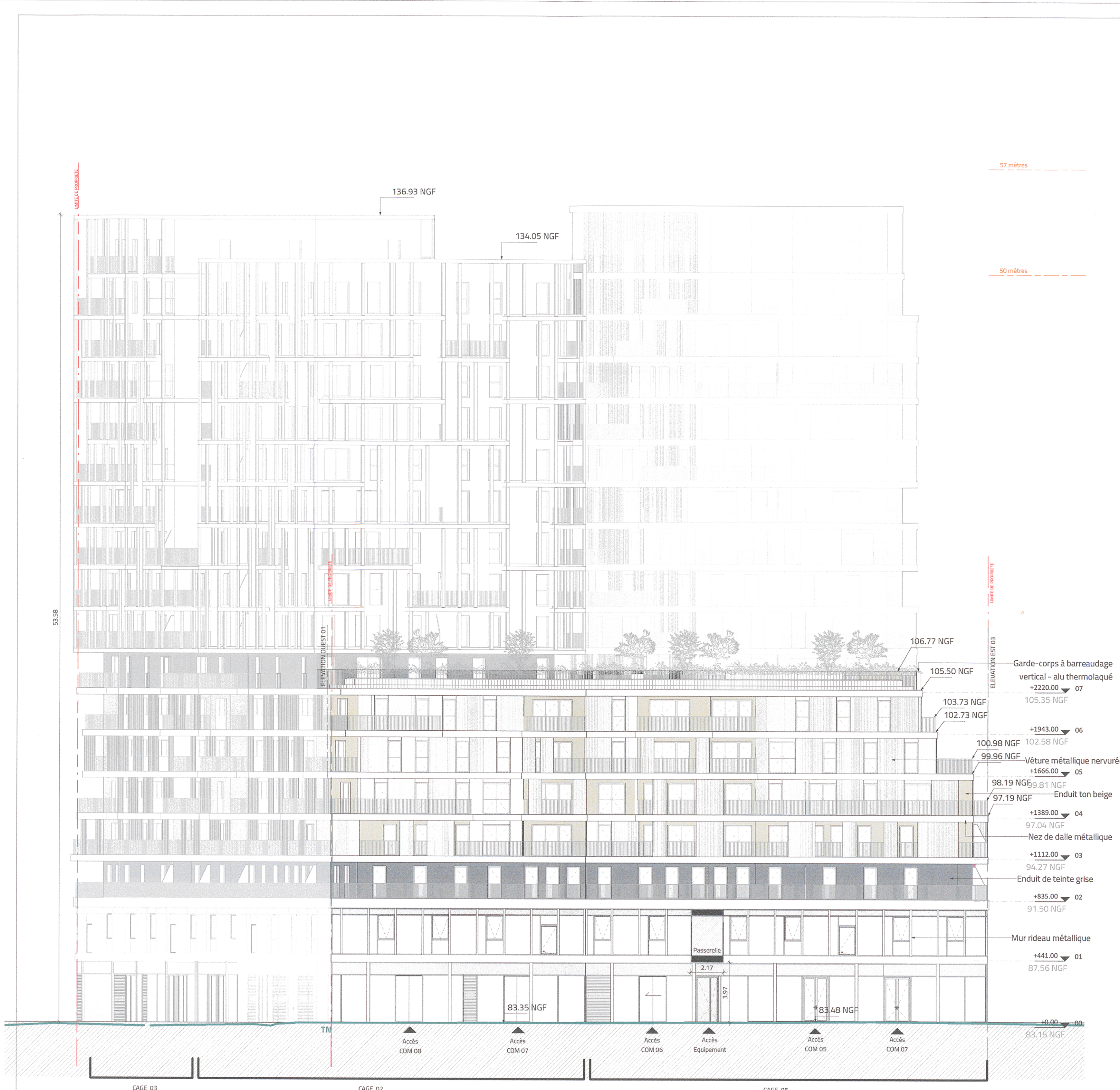
PC05a2_FACADE SUD 02 Ech : 1:200
