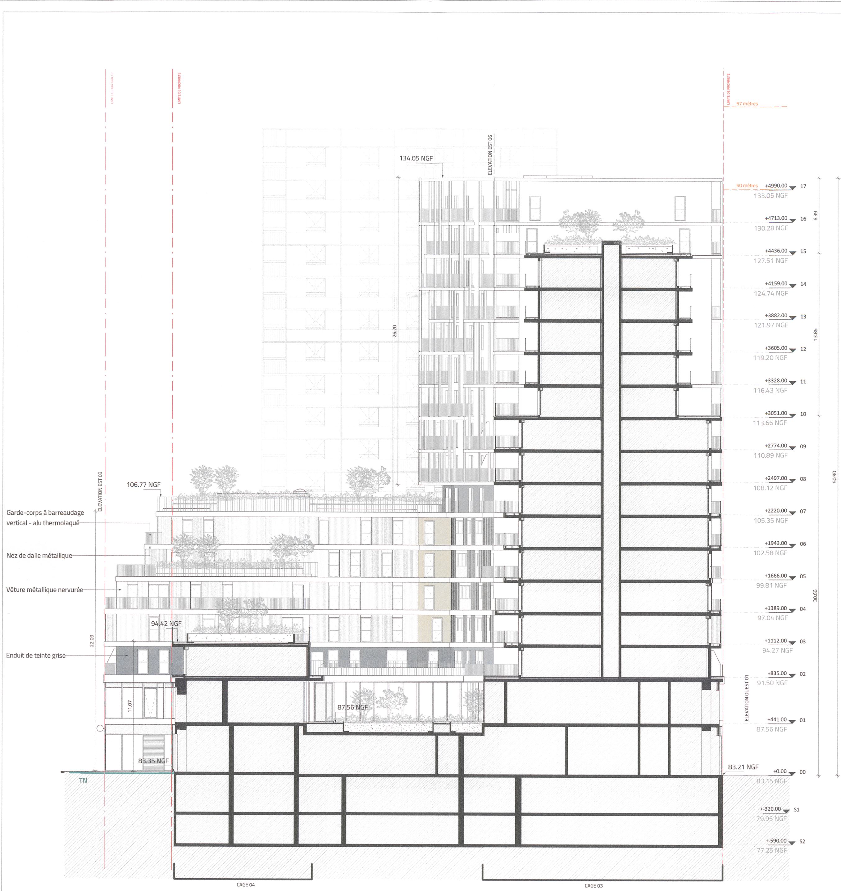
PC05b5_FACADE INTERIEURE NORD E Ech : 1 : 200
