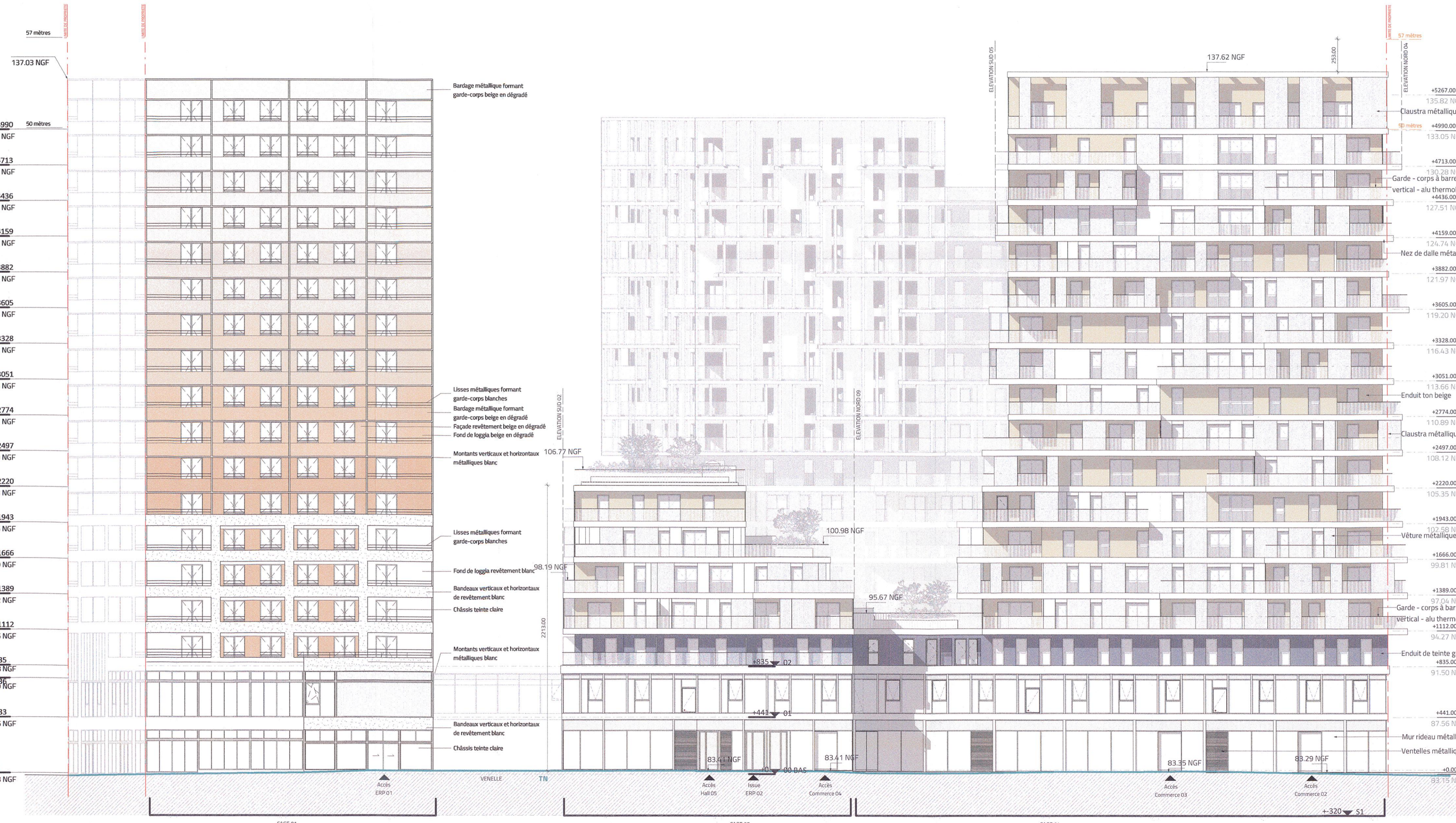
PC05a3_FACADE EST 03 Ech : 1 : 200
